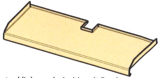
Pfostenklinkung dreiseitig mit Bord
