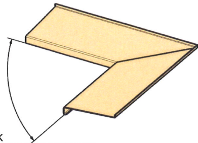
Inneneck
